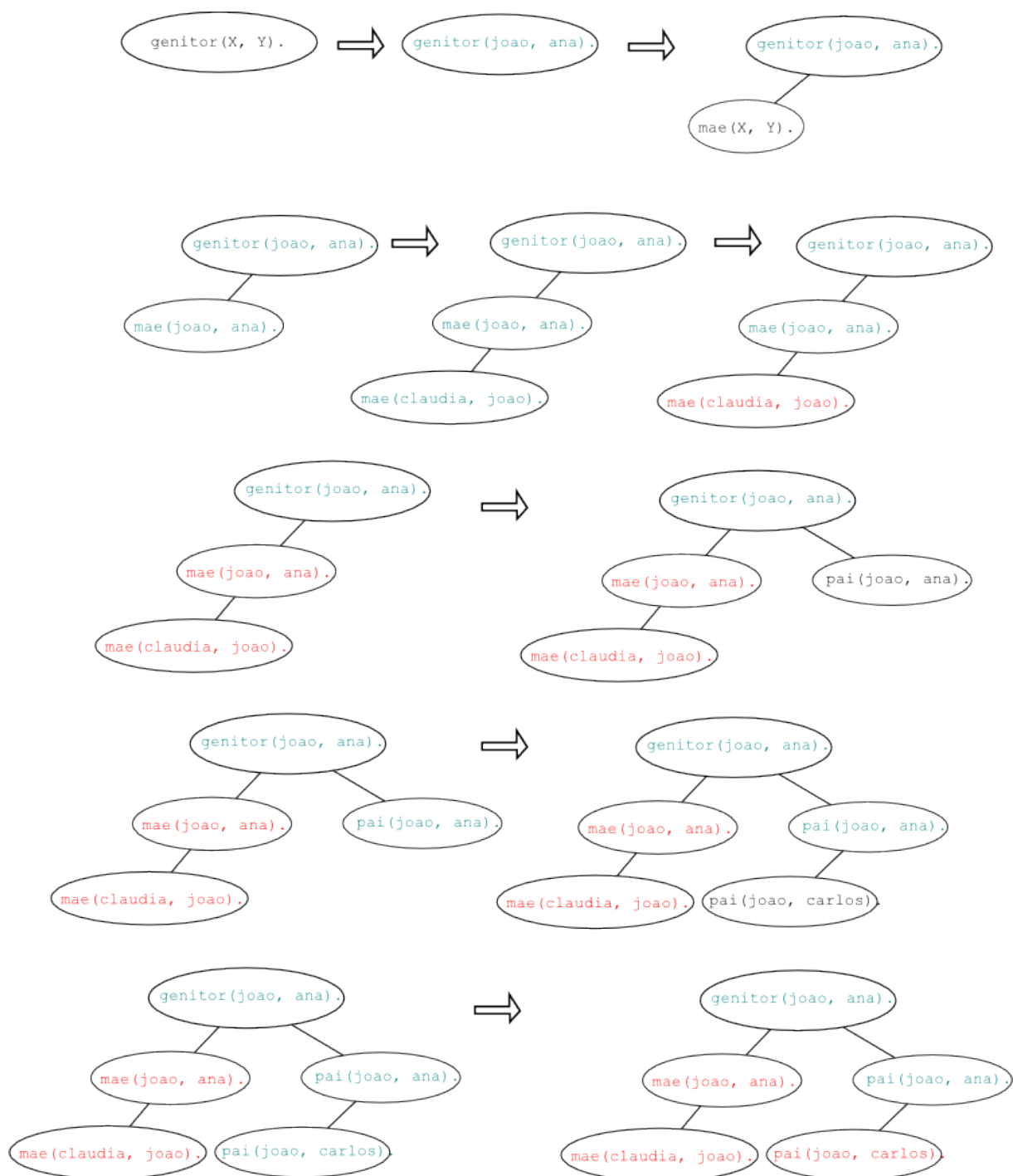
Figura 1 – Exemplo do processo de retroação realizado pelo mecanismo de inferência da linguagem Prolog.
