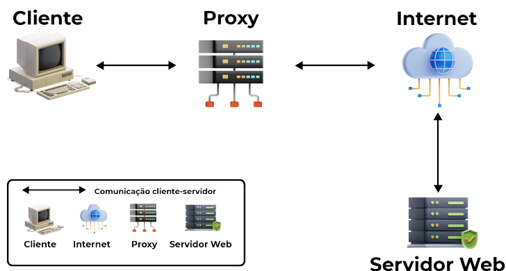
Figura 2 – Arquitetura de um servidor textitproxy.
