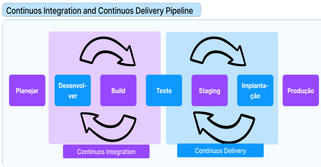
Figura 4 – CI/CD
