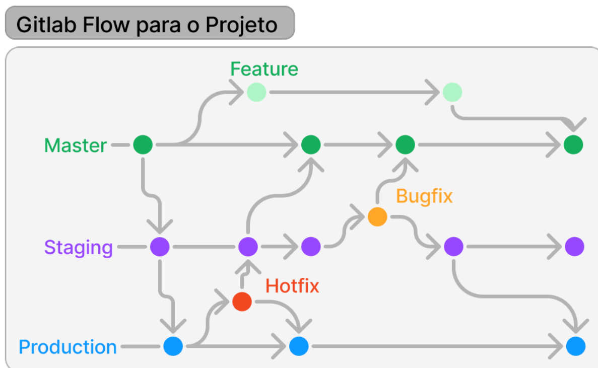
Figura 3 – Git Flow
